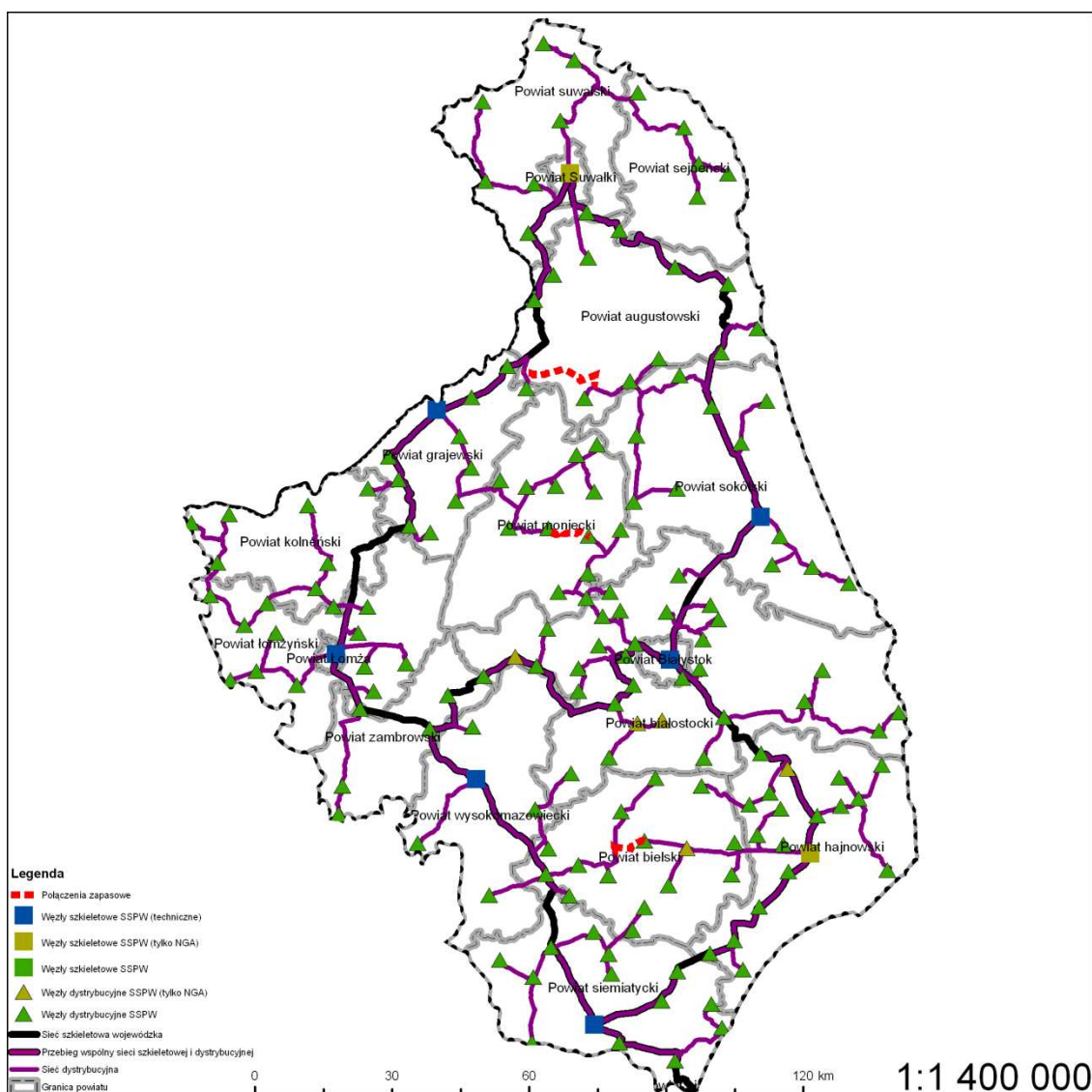
Rysunek 2 Rekomendacja rozwoju części pasywnej sieci szerokopasmowej w województwie podlaskim
